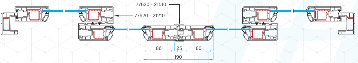
SEC A-A
