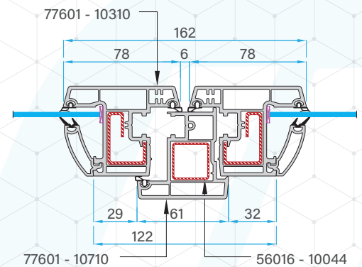
SEC A-A
