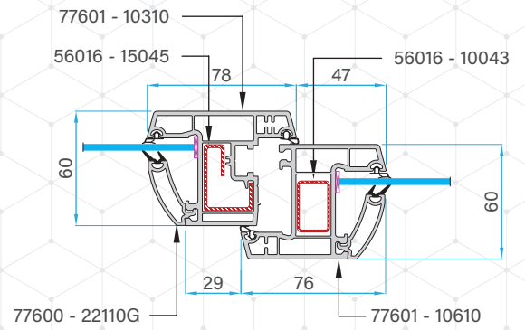
SEC A-A
