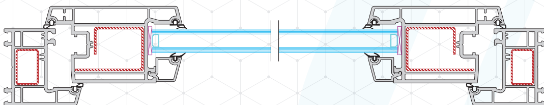
SEC A-A
