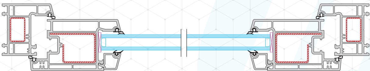
SEC A-A
