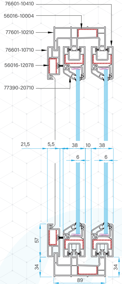
SEC-AA
