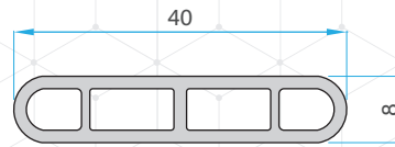
Louvre Blade 77390 - 20610
